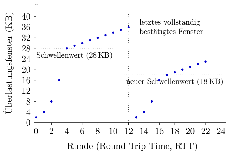
Abbildung 51: TCP Tahoe
