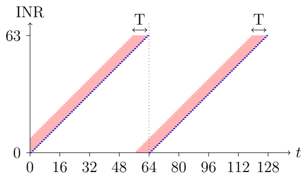
Abbildung 40: Anfangsfolgennummern
