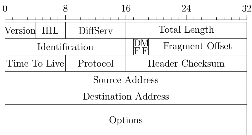
Abbildung 32: Ein IPv4-Datagramm
