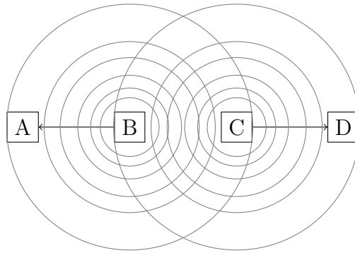
Abbildung 25: Exposed-Terminal-Problem
