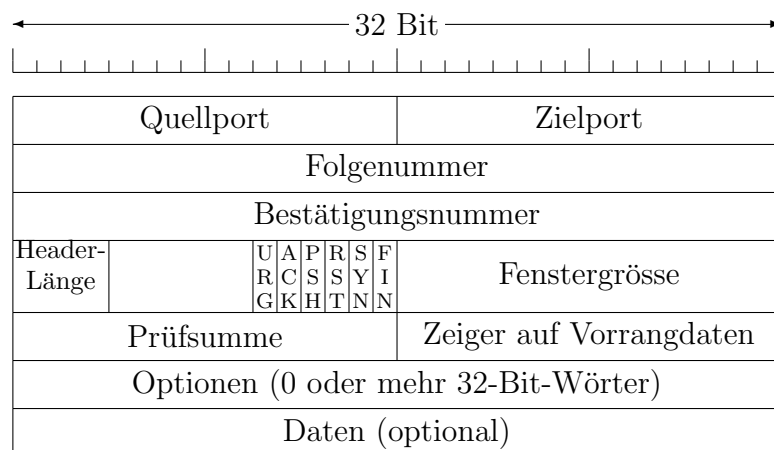
Abbildung 49: TCP-Header
