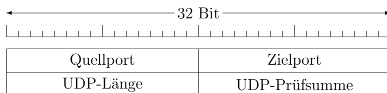
Abbildung 48: UDP-Header
