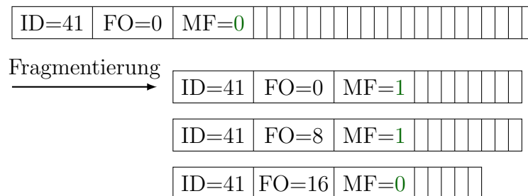
Abbildung 33: Fragmentierung
