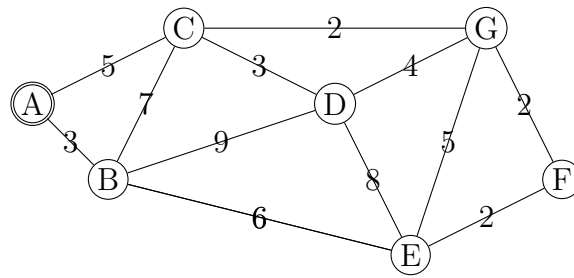
Abbildung 29: Ein Beispielgraph
