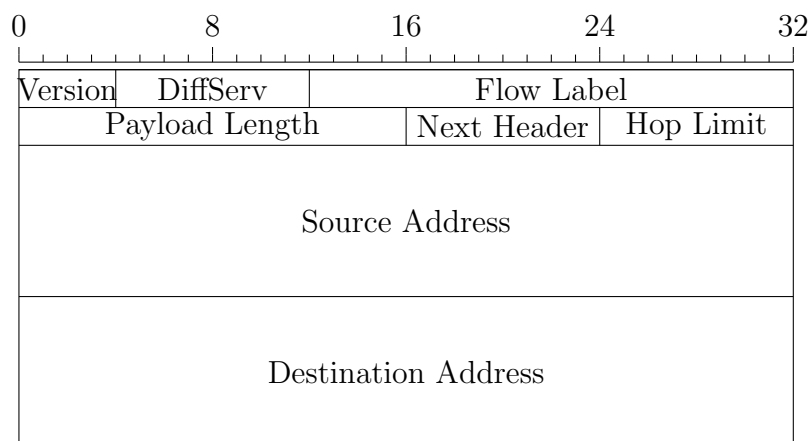
Abbildung 36: Ein IPv6-Datagramm
