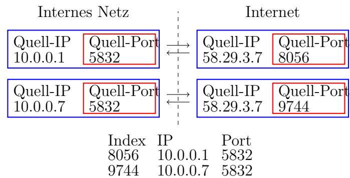
Abbildung 35: NAT
