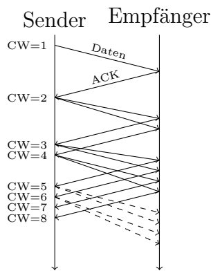
Abbildung 50: Der Slow-Start-Algorithmus
