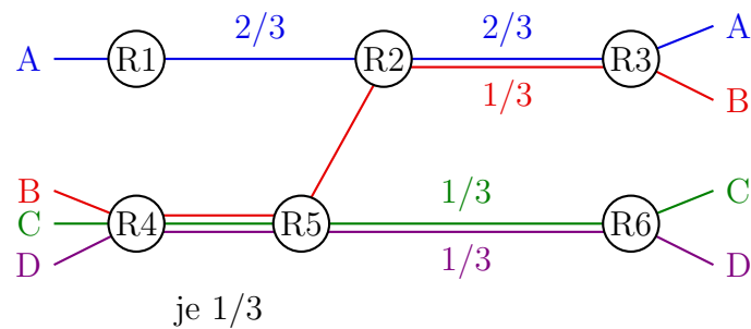
Abbildung 46: Max-Min-Zuordnung
