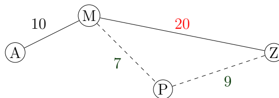
Abbildung 28: Das Optimalitätsprinzip
