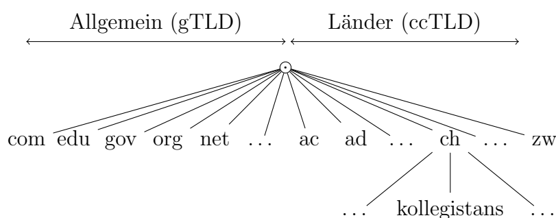
Abbildung 52: TLDs
